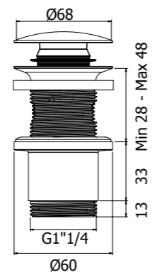
Piletta di scarico click-clack in acciaio inox, senza troppo pieno Click-clack waste unslotted, stainless steel
