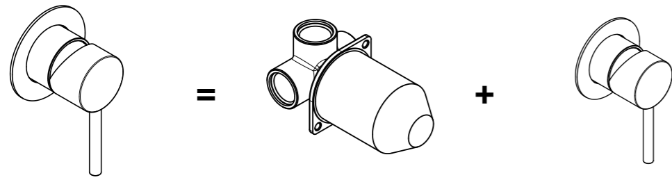
Miscelatore incasso doccia Concealed shower mixer
