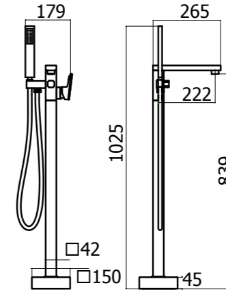
Miscelatore vasca a pavimento con kit doccia. Kit di fissaggio venduto separatamente
